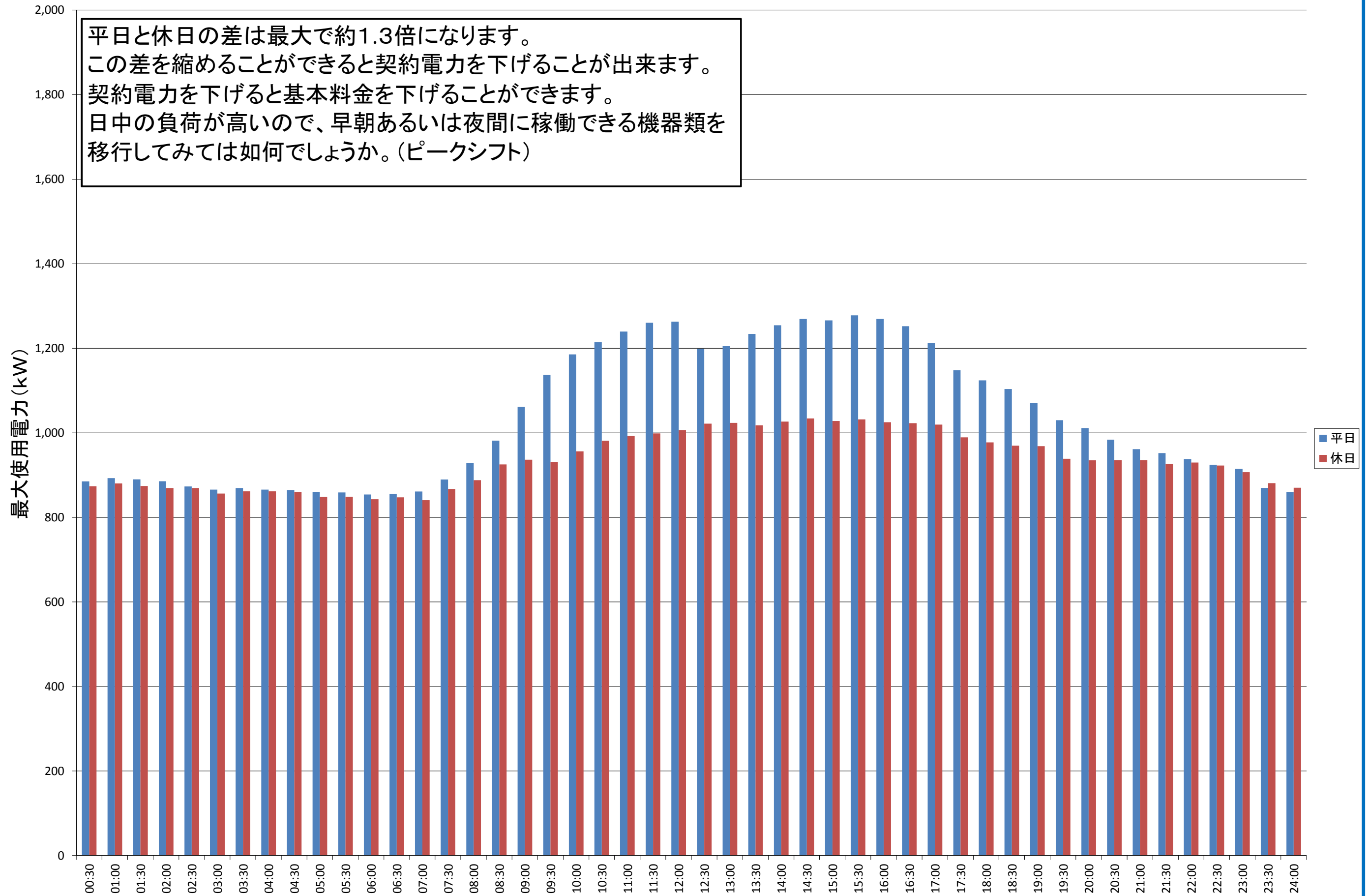
本荘中キャンパス 9月の時間帯別最大使用電力平均値
