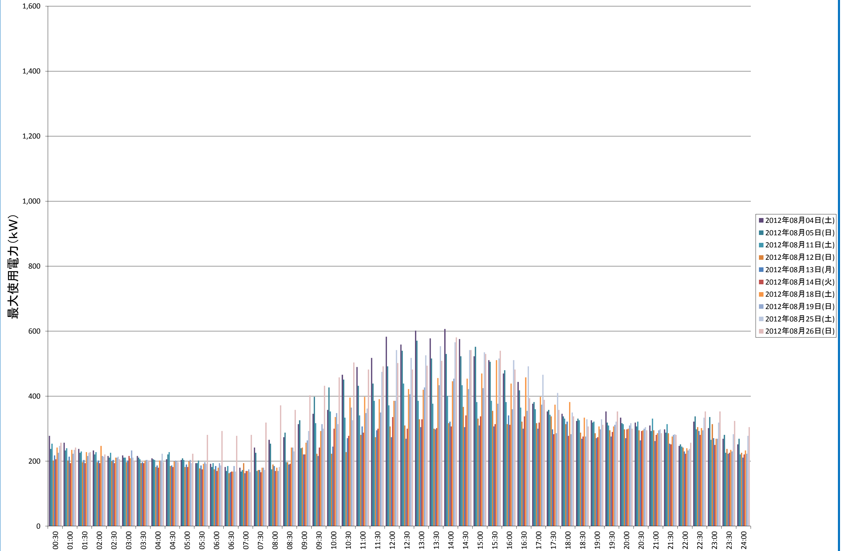
黒髪北キャンパス 8月の時間帯別最大使用電力(土日祝)
