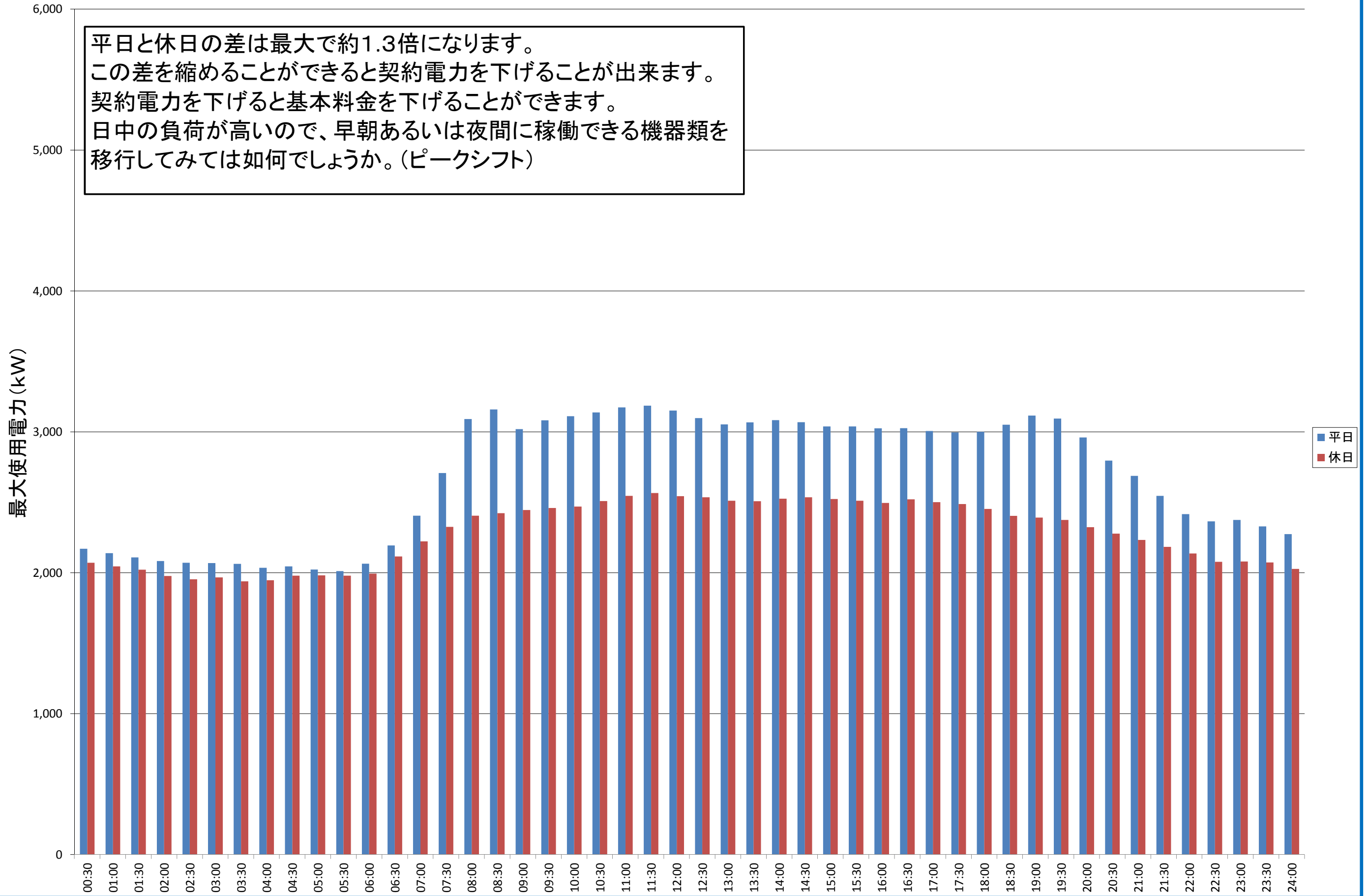
本荘北キャンパス 1月の時間帯別最大使用電力平均値
