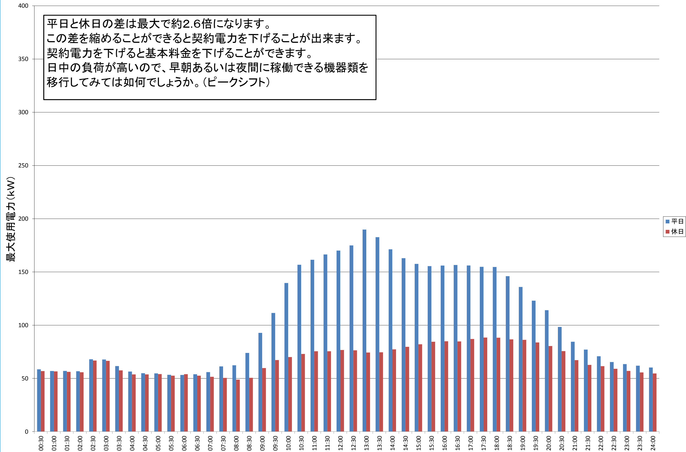
本荘南キャンパス 12月の時間帯別最大使用電力平均値
