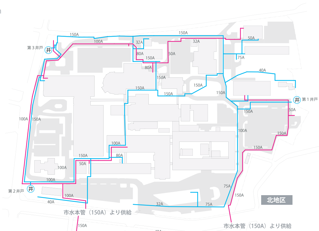
給水設備 現状 給水設備配管図
