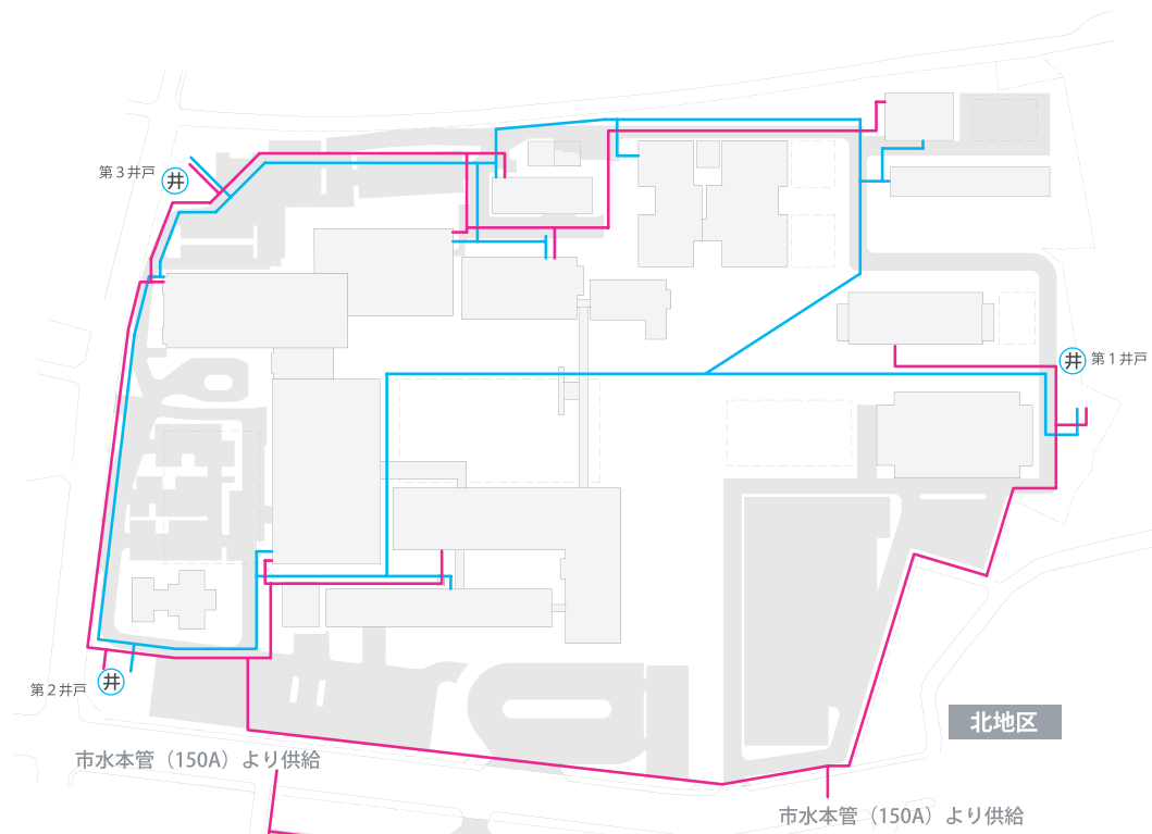
給水設備 計画 給水設備配管図
